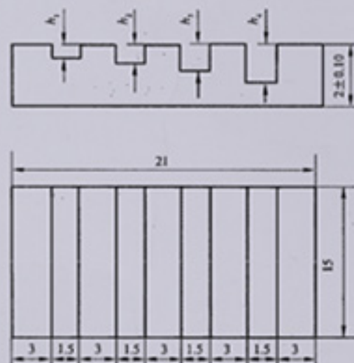
图 L.2 II型对比试块
